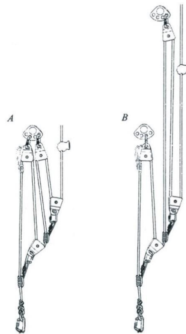
Сложный полиспаст 9:1
