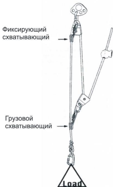
Простой полиспаст 3:1 из грузовой веревки
