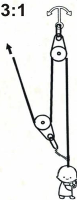
Простые полиспасты 2:1 и 3:1
