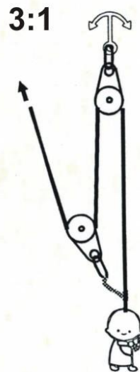
Простые полиспасты 2:1 и 3:1
