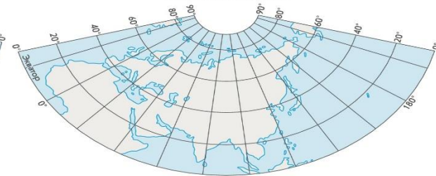
РАВНОВЕЛИКАЯ
