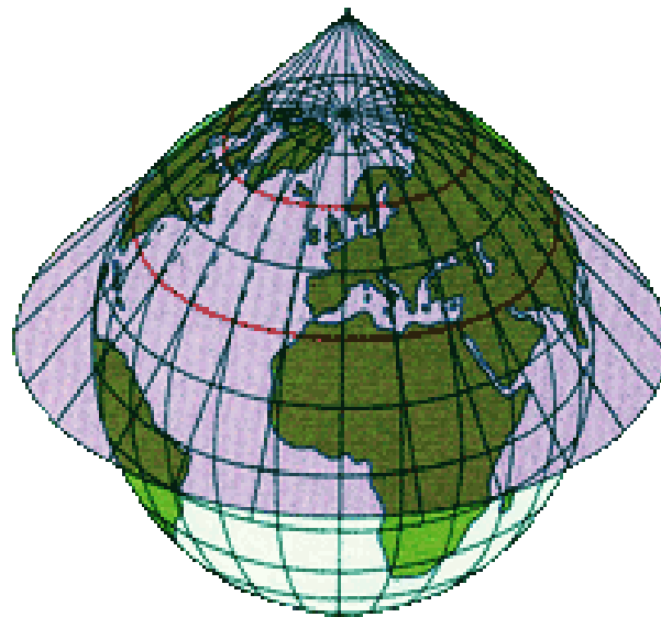
Коническая
