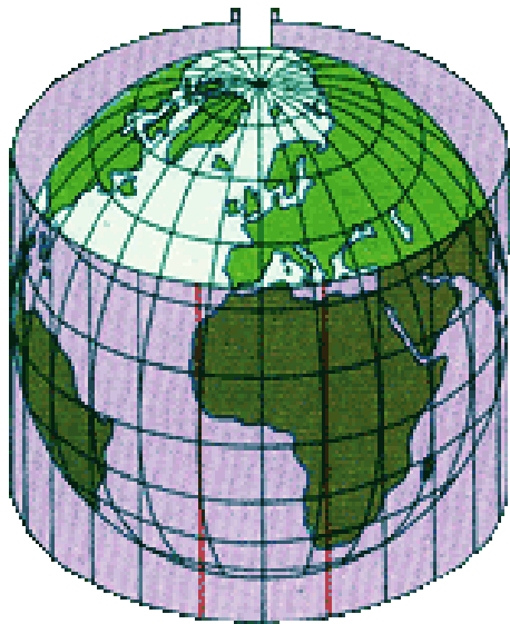
Цилиндрическая
