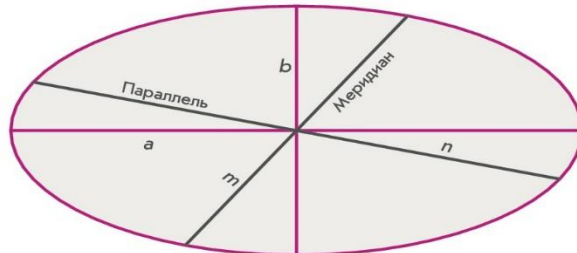
ЭЛЛИПС ИСКАЖЕНИЙ
