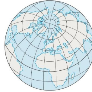
КОСАЯ РАВНОВЕЛИКАЯ
