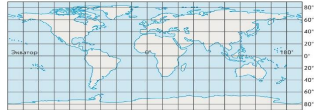
РАВНОПРОМЕЖУТОЧНАЯ
