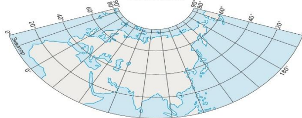
РАВНОВЕЛИКАЯ
